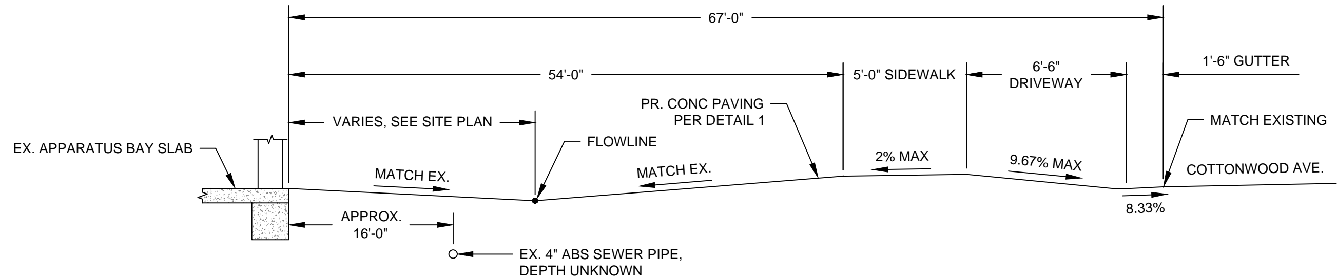
SECTION VIEW "A" SCALE: N.T.S.
