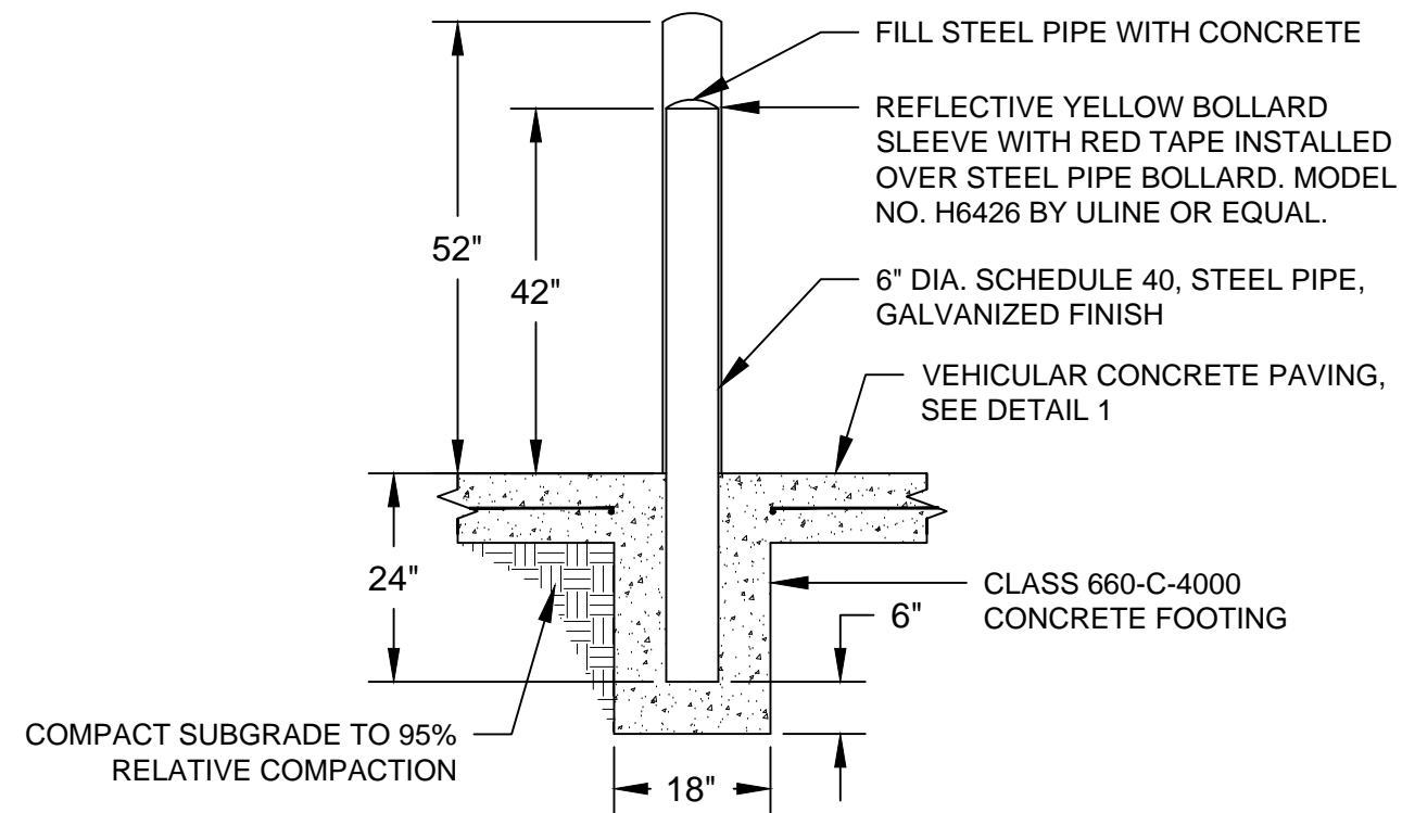
STEEL PIPE BOLLARD SCALE: 1/2" = 1'
